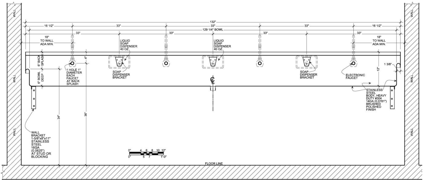
SECTION: LONGITUDINAL
