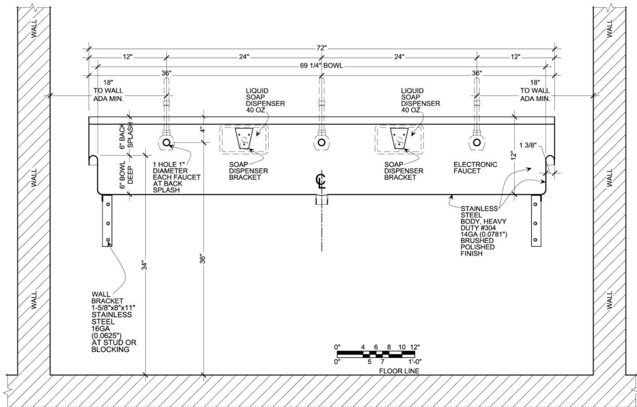
SECTION: LONGITUDINAL
