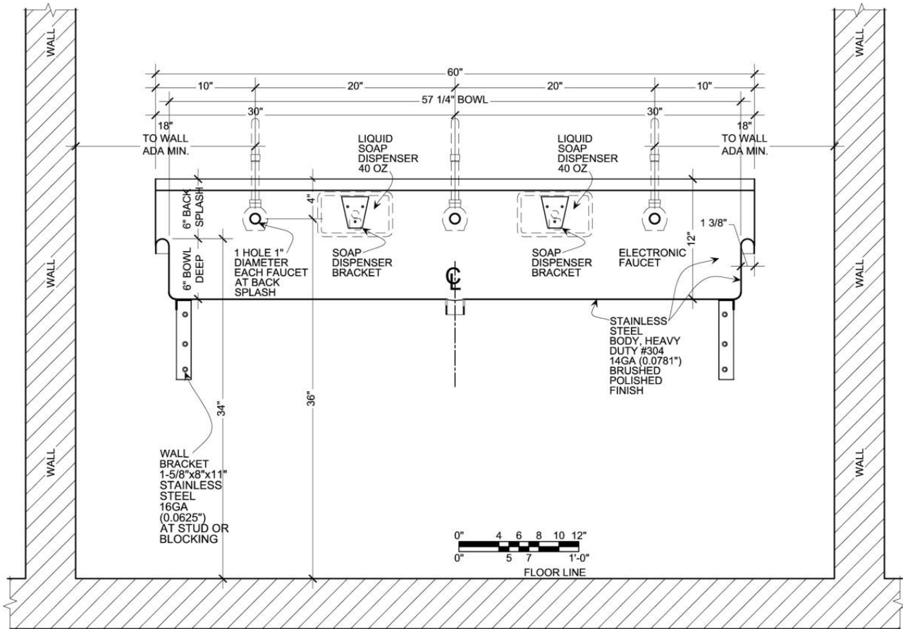
SECTION: LONGITUDINAL
